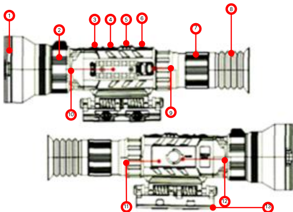
Рис. 1. Устройство прицела
